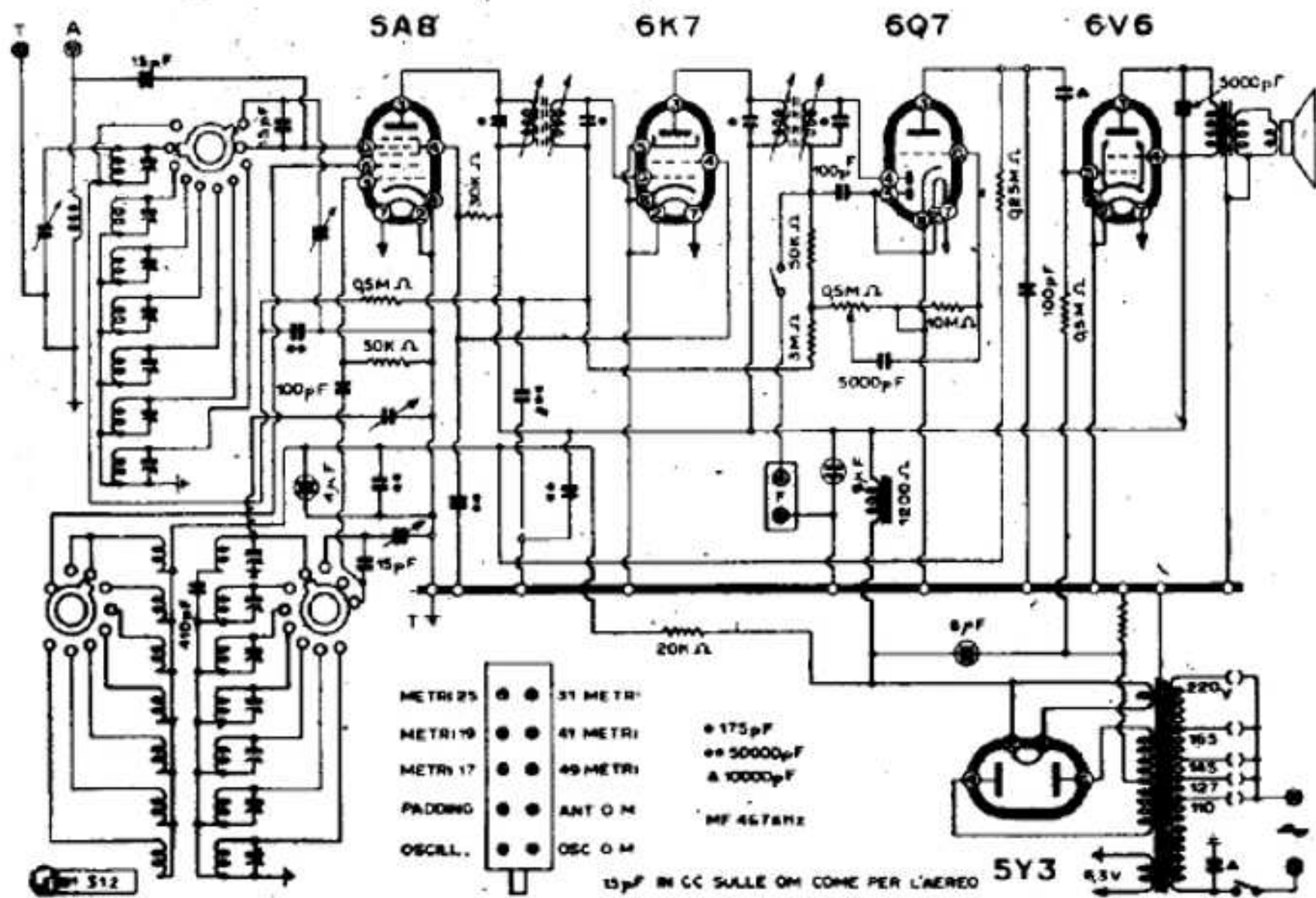
AREL - MODD. « ARELVOX I » - « ARELVOX II »
